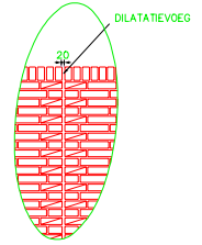
DETAIL METSELWERK EN VOEG SCHAAL 1 : 20
