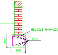
AANZICHT KOPSEKANT SCHAAL 1 : 20
