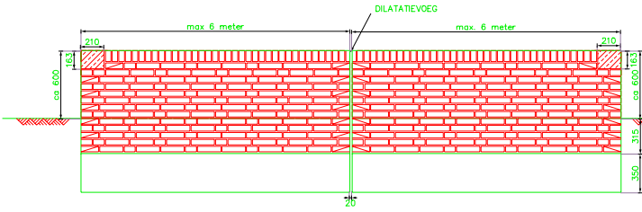
LAGE MUUR OP STAAL SCHAAL 1 : 20
